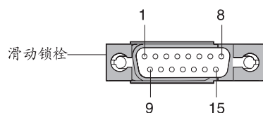
图 4-13. 型号为 016 的以太网台式集线器 AUI 端口
