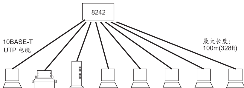
图 4-3. 用单个型号 008 构建一个 10BASE-T 网络
