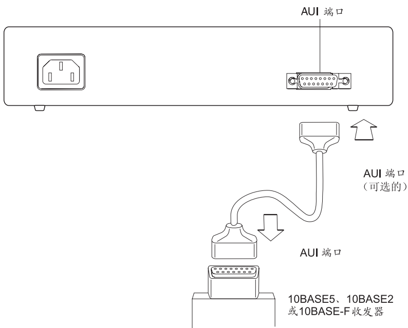
图 2-5. 连接 AUI 电缆(型号 016)
